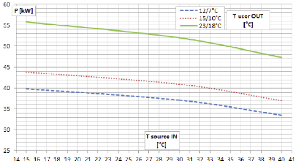
XE 33 – Potenza assorbita in raffreddamento al variare della temperatura lato sorgente
