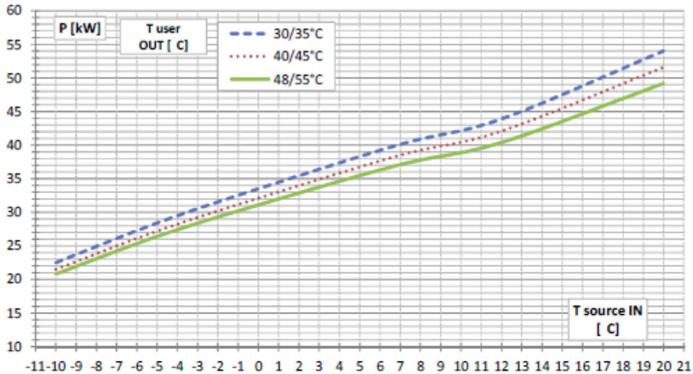
XE 33 – Potenza assorbita in riscaldamento al variare della temperatura lato sorgente
