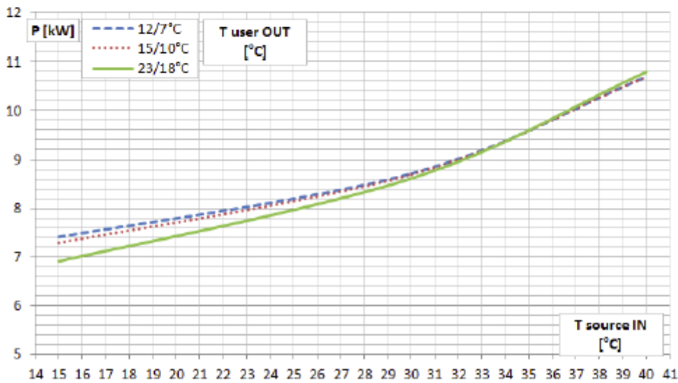
XE 33 – Potenza assorbita in raffreddamento al variare della temperatura lato sorgente
